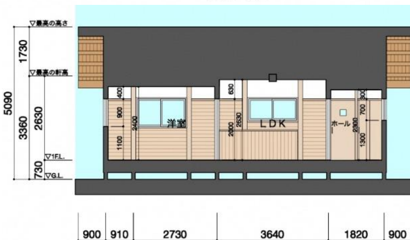
南側立面図
