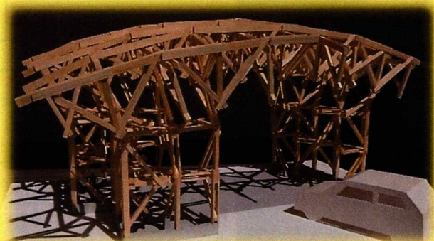
現場見学会において見学する『モックアップを兼ねたゲート』
