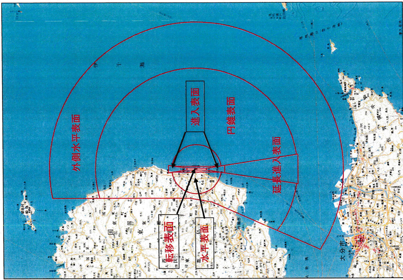
大分空港の制限表面区域図
